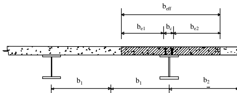
Figura 7.4 - Definizione della larghezza efficace b_{eff} e delle aliquote b_{ci} .
